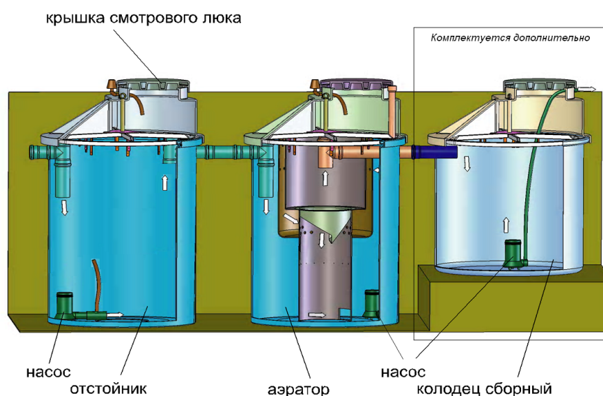
Рис. 3 Установка Aquatech ЛОС 8А
