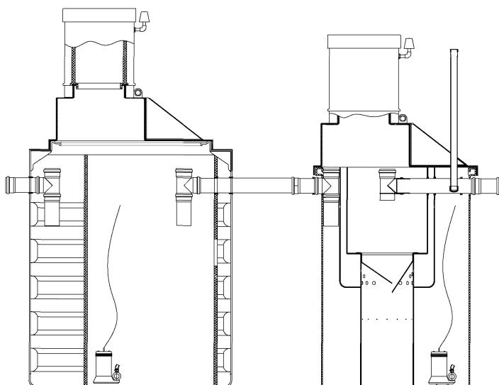
Рис. 4 Установка Aquatech ЛОС 15
