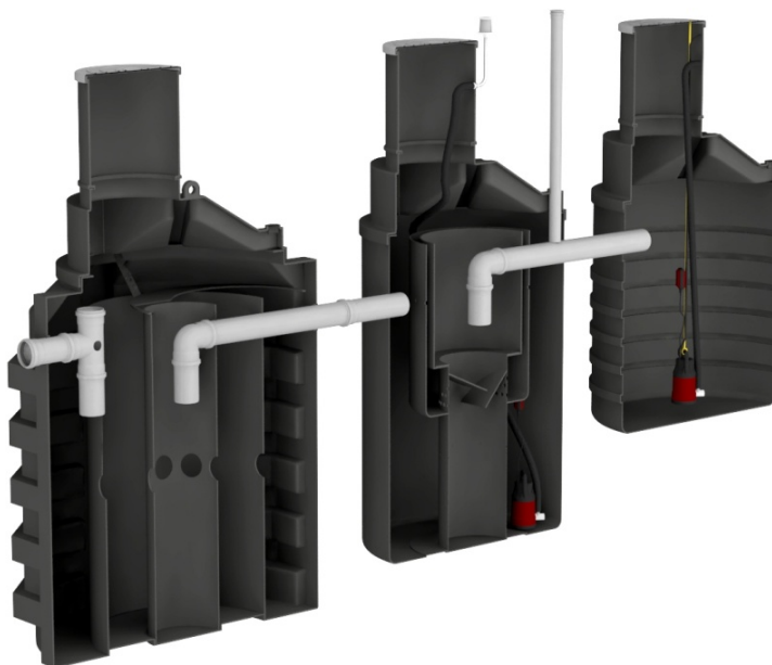
Рис. 1 Установки Aquatech ЛОС 5, ЛОС 8
